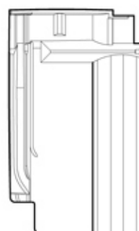
Țiglă de închidere sub coamă laterală dreapta
